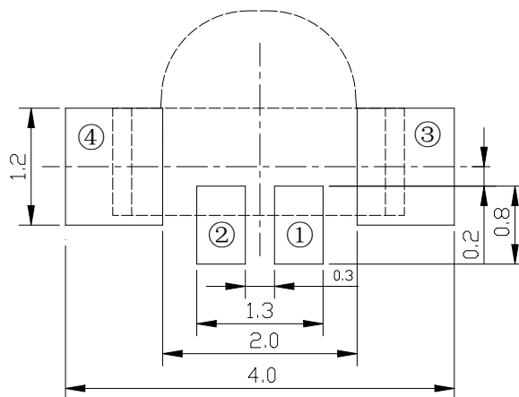
推荐焊盘尺寸
